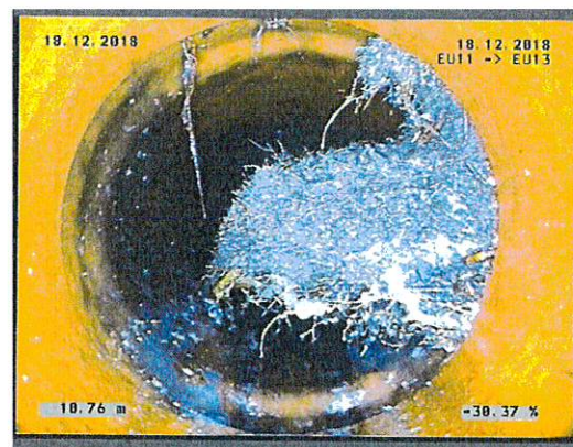
Figure 4: Introduction de racine dans le collecteur EU
